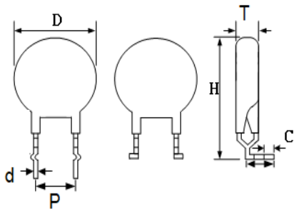
T 型 (前后弯脚+90°弯折+外弯)
